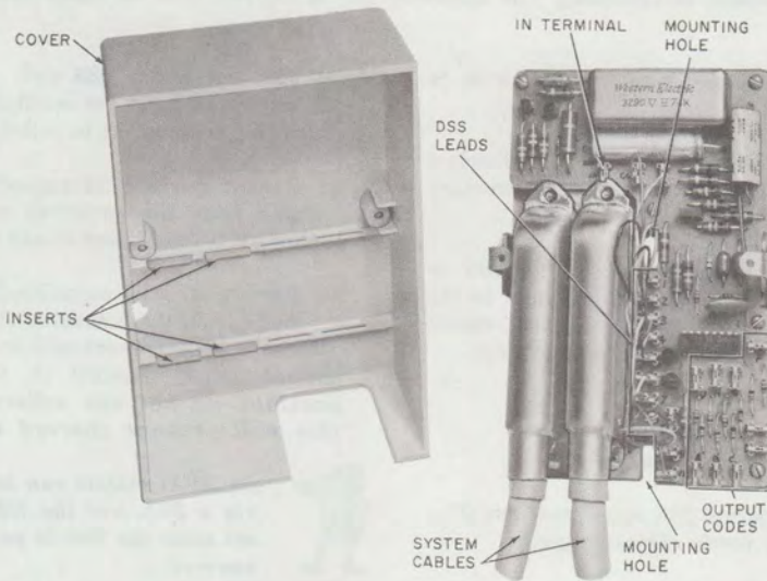
Fig. 35-26A Apparatus Unit
