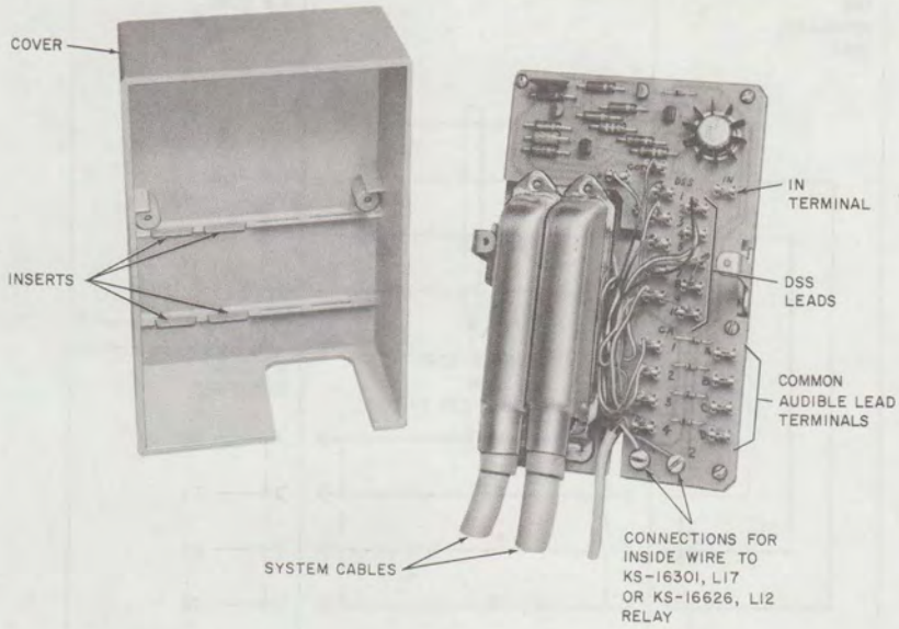
Fig. 34-25A Apparatus Unit
