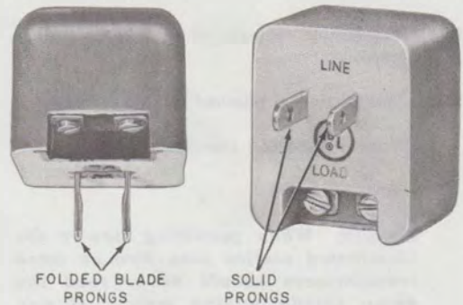
Fig. 2—2012-Type Transformer, Prongs
