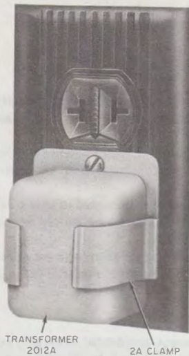
Fig. 1—2A Clamp
