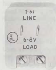
Fig. 4—2012A Transformer
