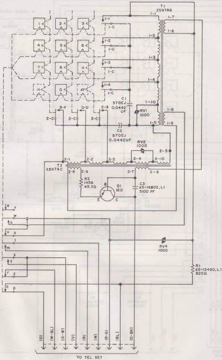
Fig. 20—2553 Dial, Schematic
