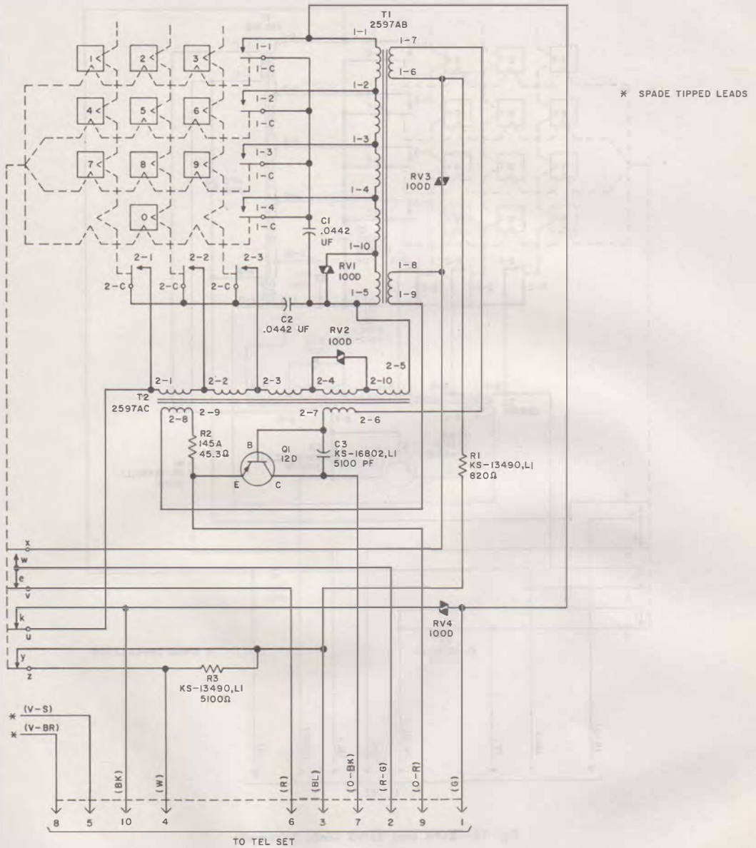
Fig. 17—2513 Dial, Schematic
