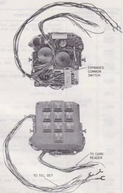
Fig. 6—25R3 Dial
