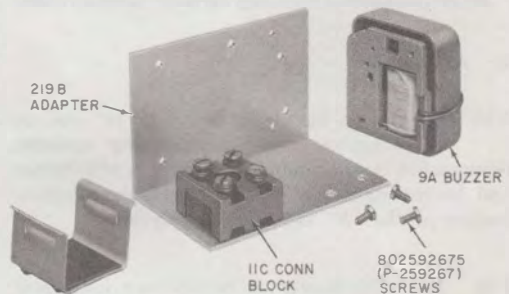
Fig. 4—9B Buzzer
