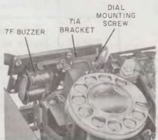
Fig. 15—71A Bracket
